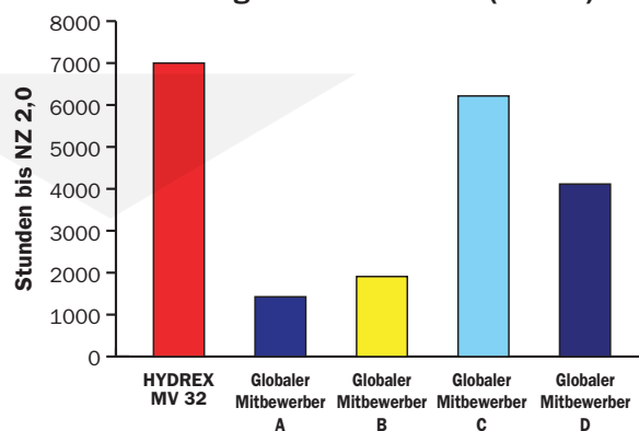
Vergleich der Oxidationsdauer Prüfung nach ASTM D943 (ISO 32)
